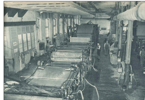
Atpūta, Nr. 7 (07.02.1941). Galvenā mašīna, kas papīru putru pārvērš pergaminā
